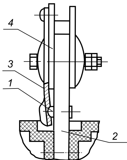
1 - сферический упор; 2 - неподвижный контакт; 3 - пружинная пластина; 4 - подвижный контакт.
